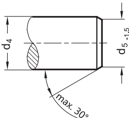
轴详图
